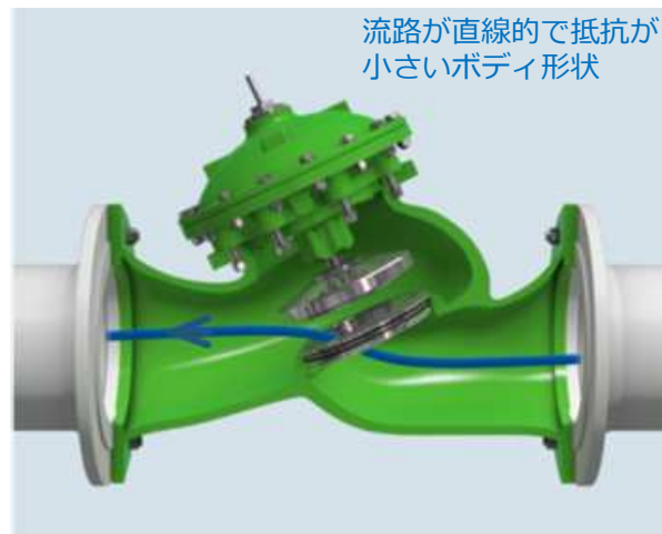
当社Y型ボディー
