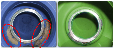
キャビテーション発生によるバルブ損傷例
