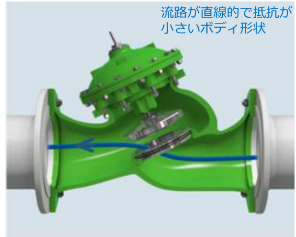
当社Y型ボディ
